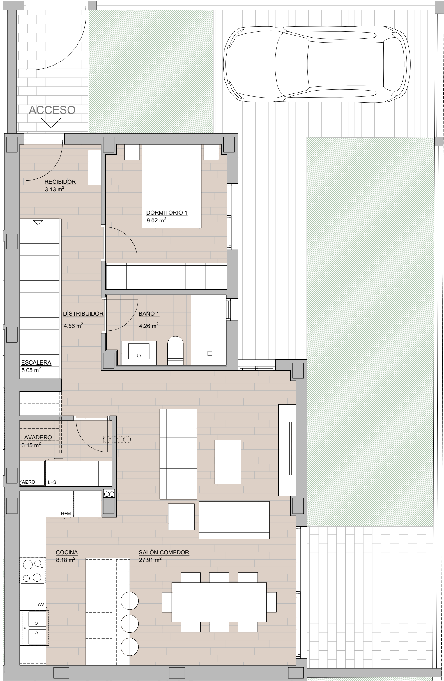
PLANTA BAJA
